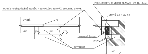
NOVÝ STAV - PŮDORYS A ŘEZ
