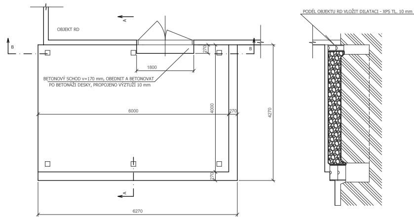
NOVÝ STAV - PŮDORYS A ŘEZY
