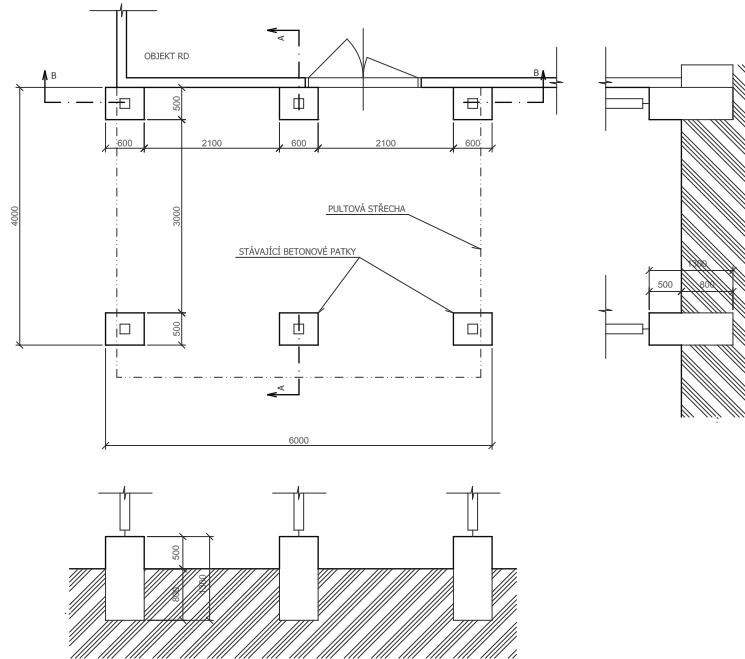
STÁVAJÍCÍ STAV - PŮDORYS A ŘEZY
