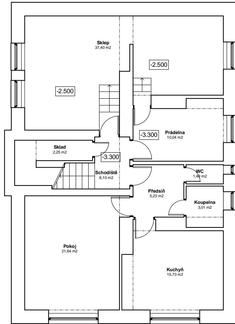
STÁVAJÍCÍ STAV 1:100
