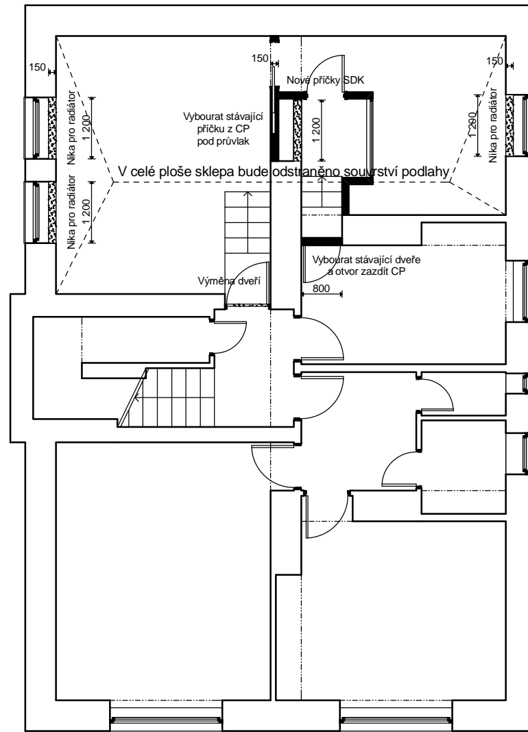
BOURACÍ PRÁCE 1:100
