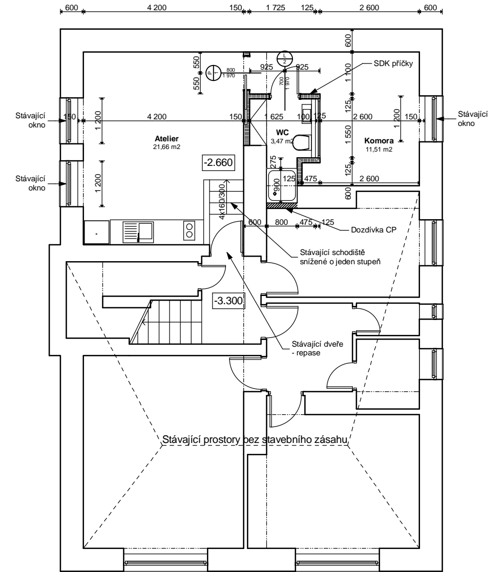
NÁVRH 1:100
