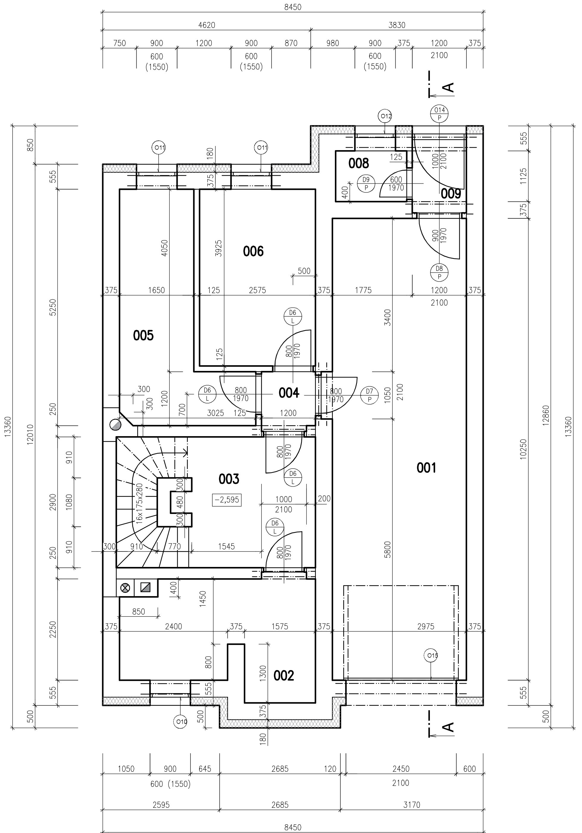
RD LILIOVÁ 415 – NAVRHOVANÝ STAV – 1.PP
