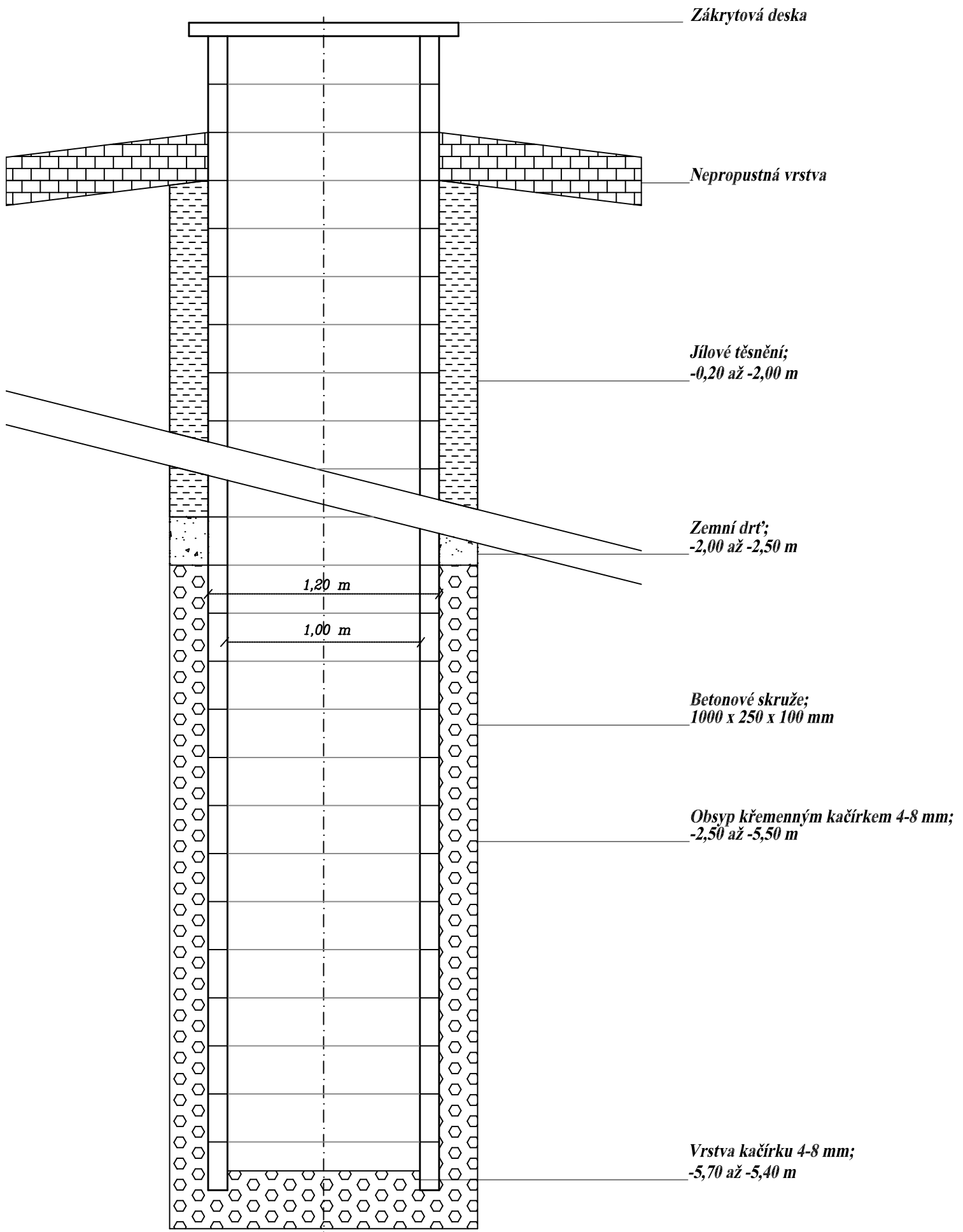
Př.č. 5 - Konstrukce studny
