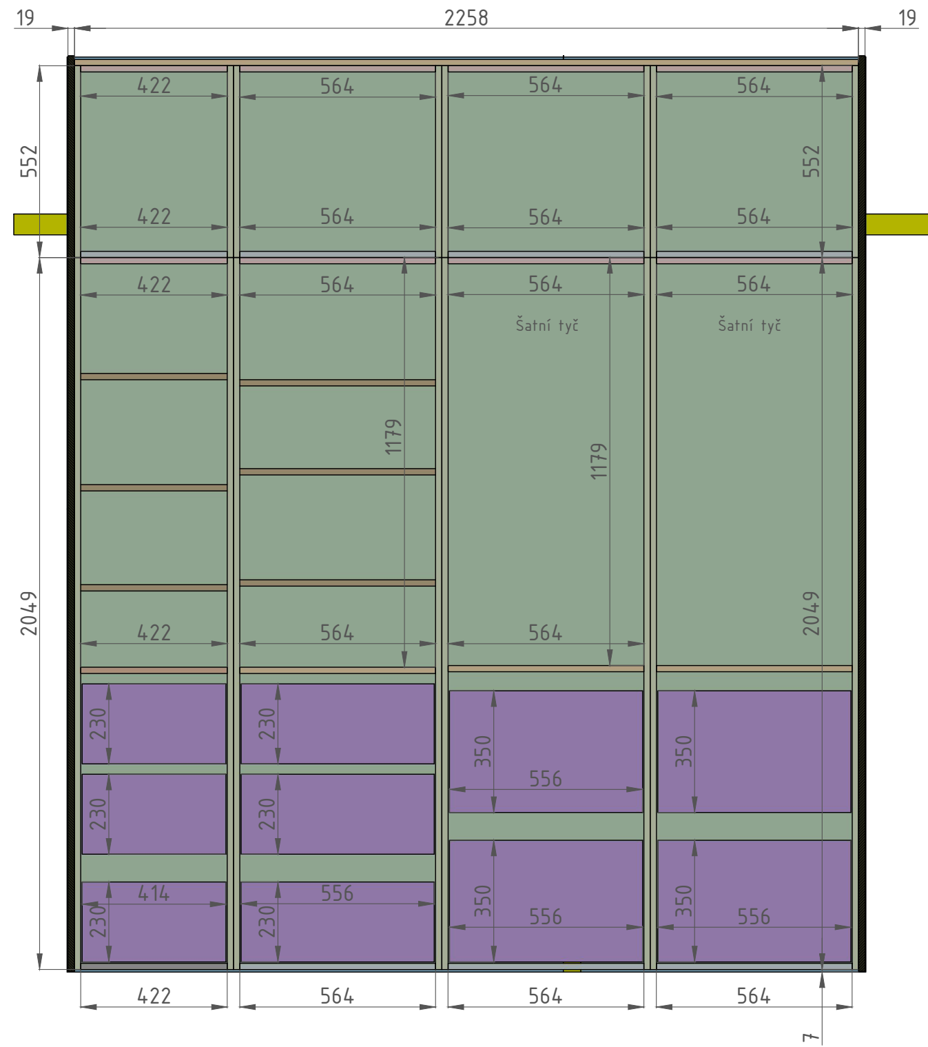
B-B (1:15)
