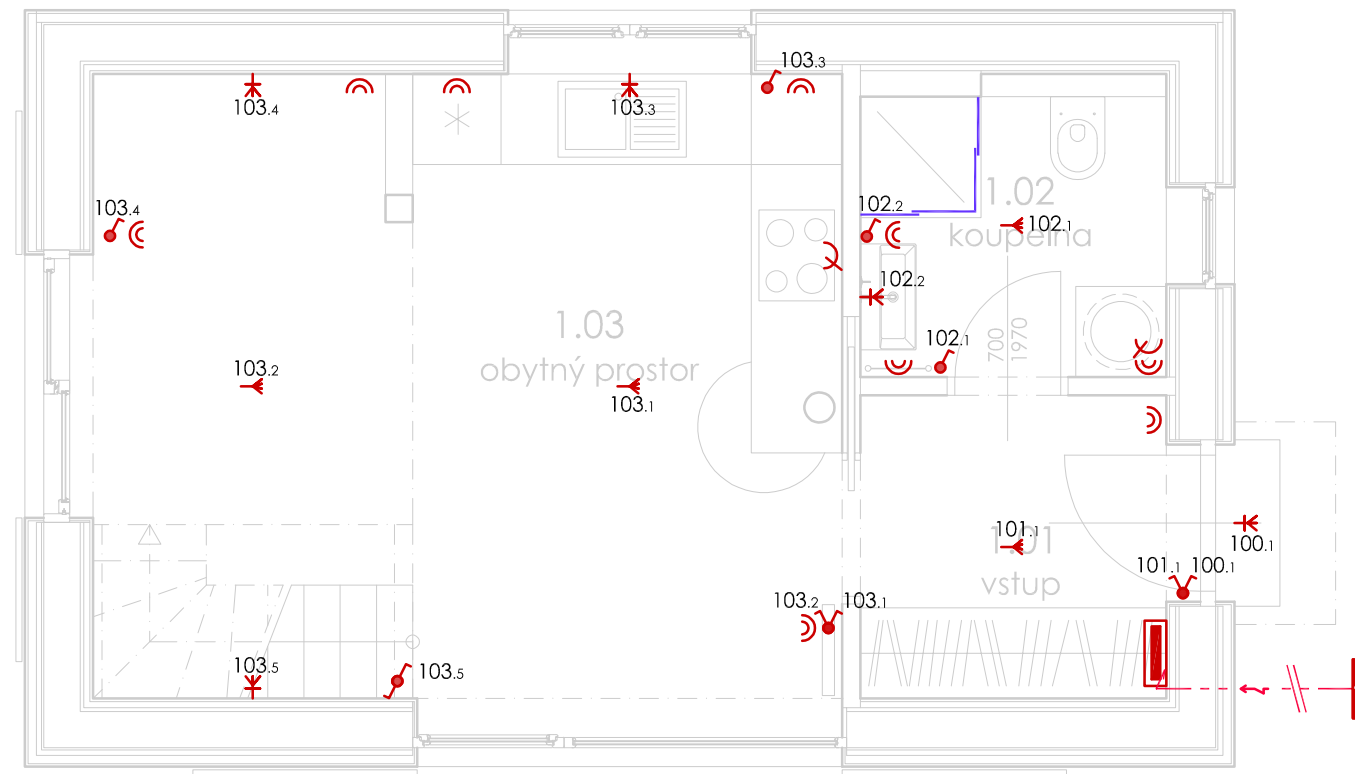
PŮDORYS 1.NP
