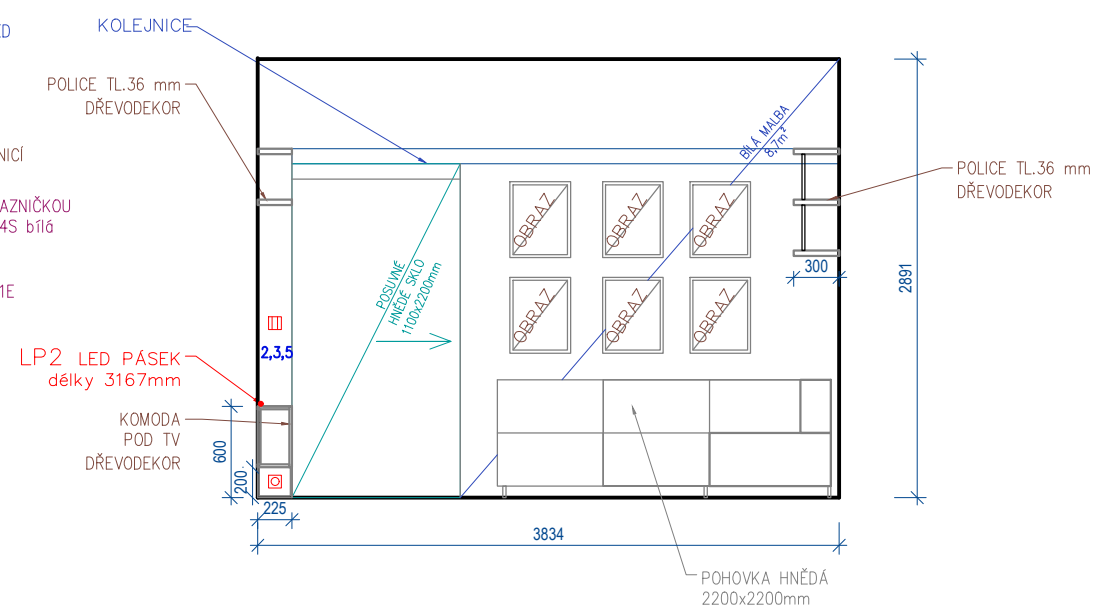
POHLED D
