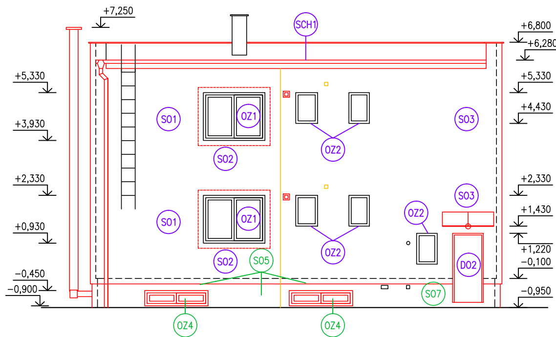
POHLED JIHOZÁPADNÍ
