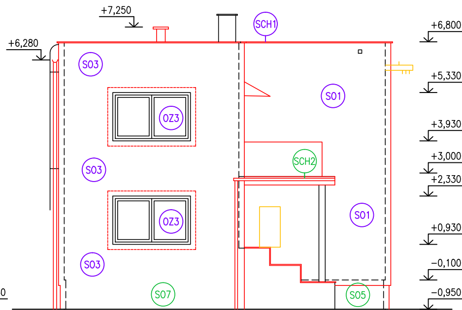
POHLED JIHOVÝCHODNÍ
