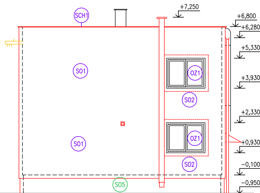
POHLED SEVEROZÁPADNÍ
