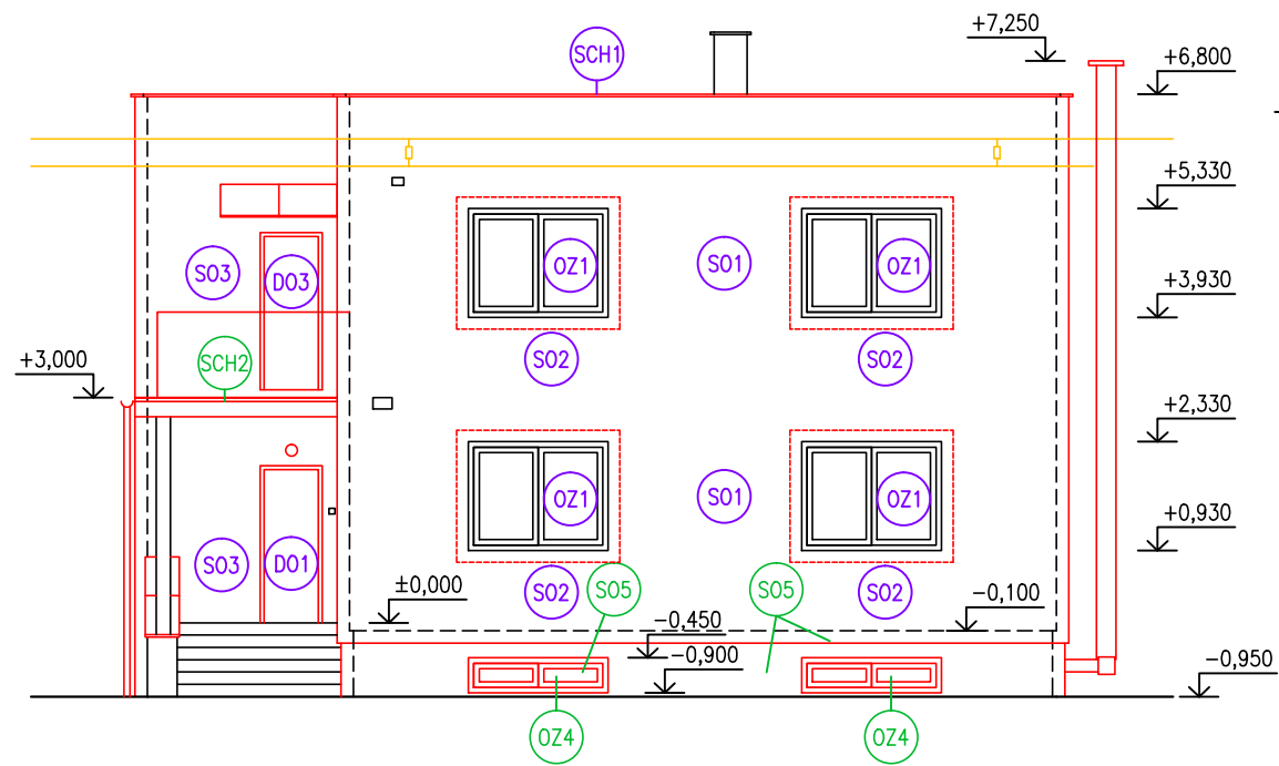
POHLED SEVEROVÝCHODNÍ
