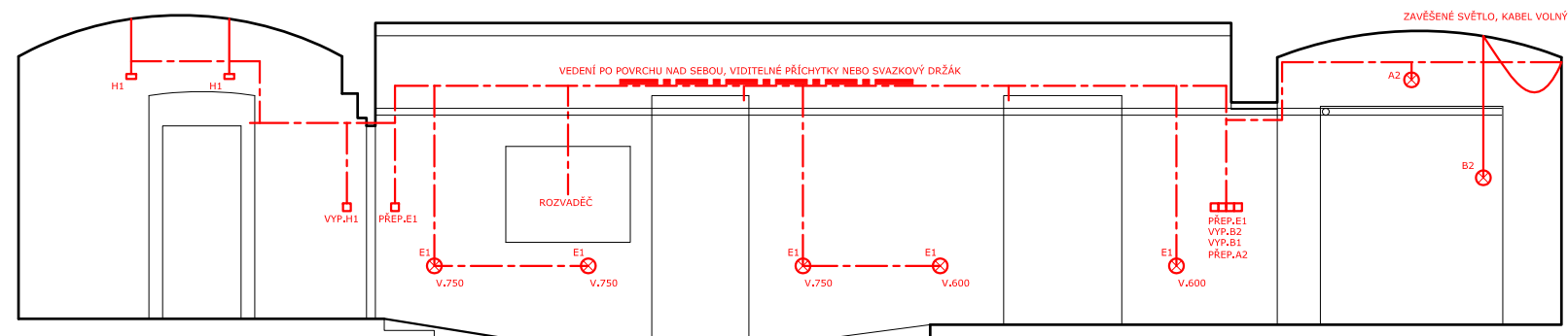
SCHÉMA ELEKTRO - ŘEZ CHODBA KUCHYNĚ 13.5.2019
