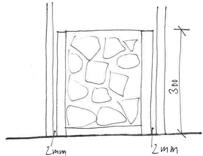
DETAIL STÍNOVÉ ŠPÁRY
