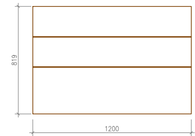
ČELNÍ POHLED - ZAVŘENÝ STAV M 1/20
