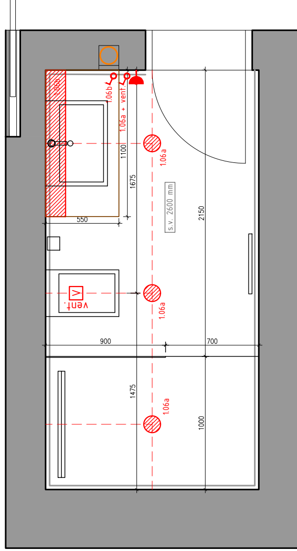
PŮDORYS
