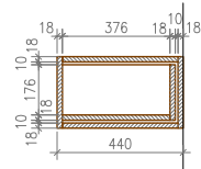
ŘEZ A-A KORPUS M 1/20
