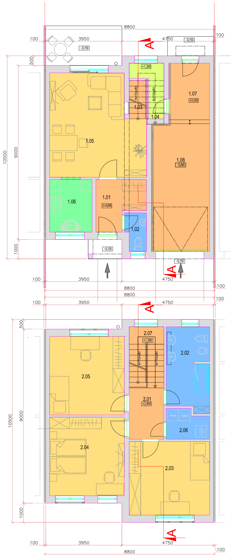
LEGENDA MÍSTNOSTÍ
