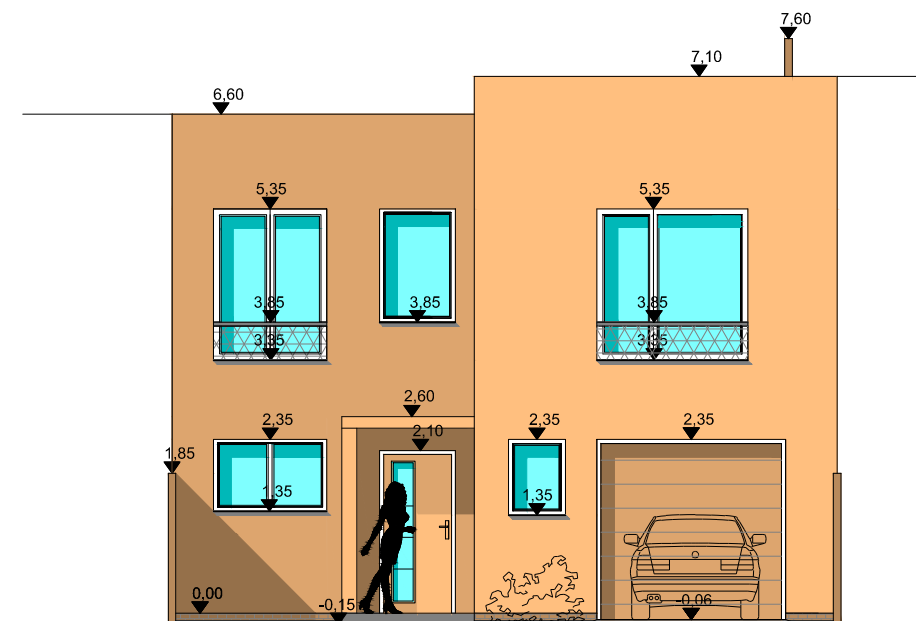
POHLED Z ULICE
