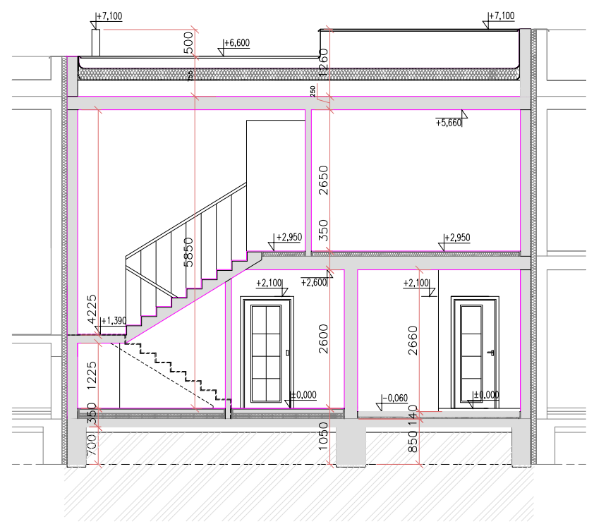
ŘEZ A-A
