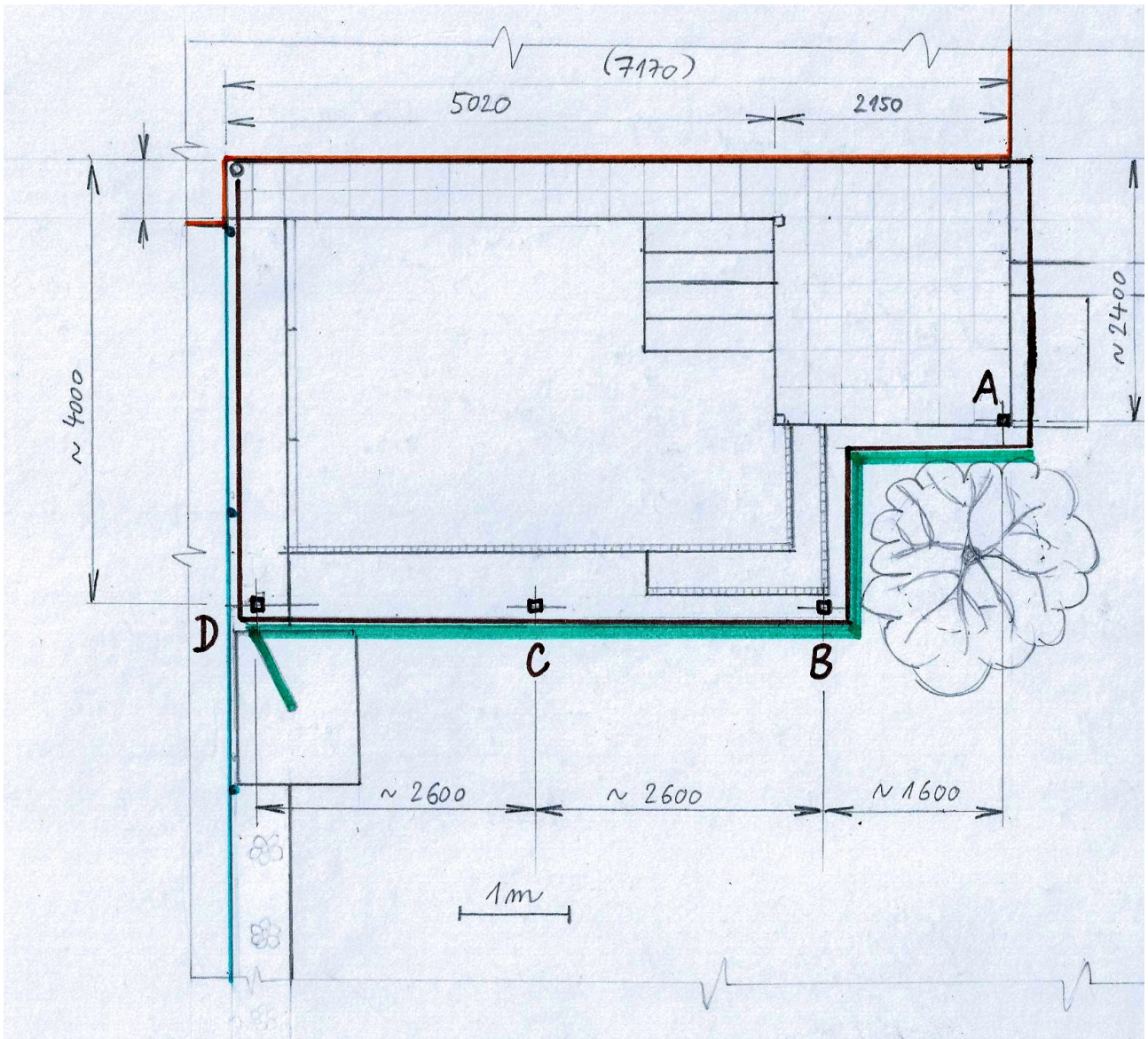
Ilustrace 1: Náčrt pergoly - půdorys
