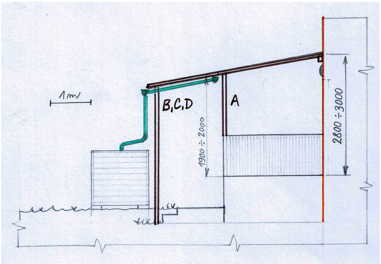
Ilustrace 2: Náčrt pergoly - bokorys
