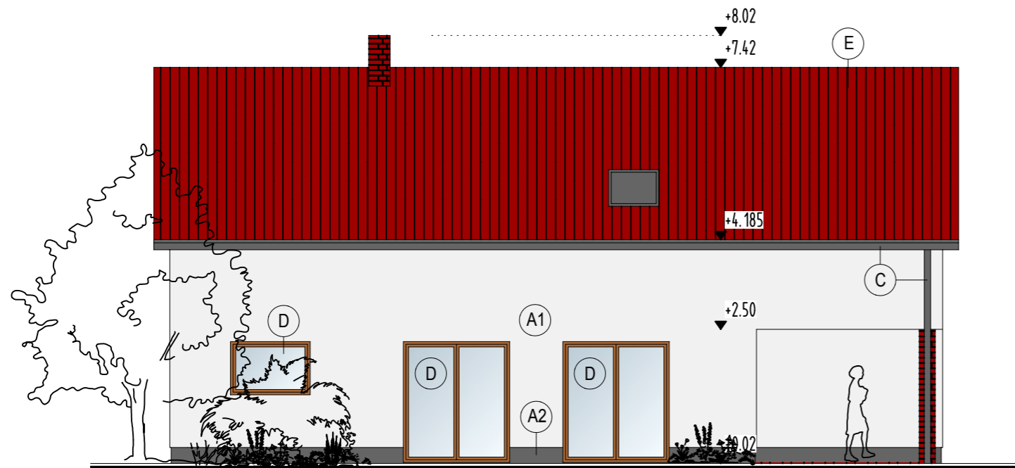
POHLED VÝCHODNÍ
