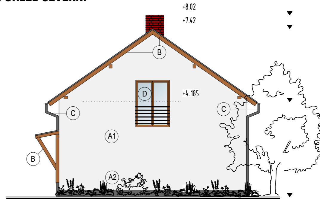
POHLED JIŽNÍ
