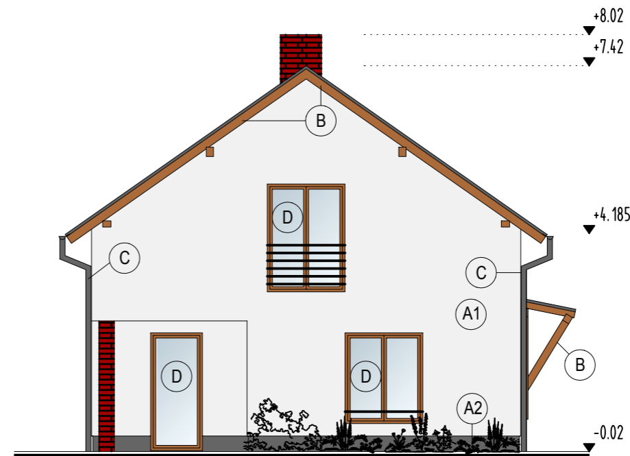
POHLED SEVERNÍ
