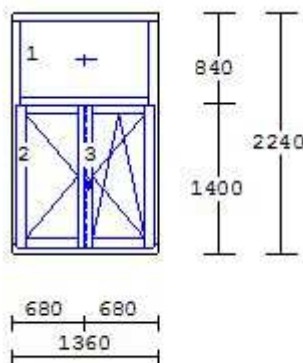
Obrázek 1: Rozměry poptávaných oken
