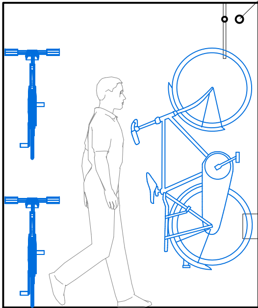
ŘEZ B-B
