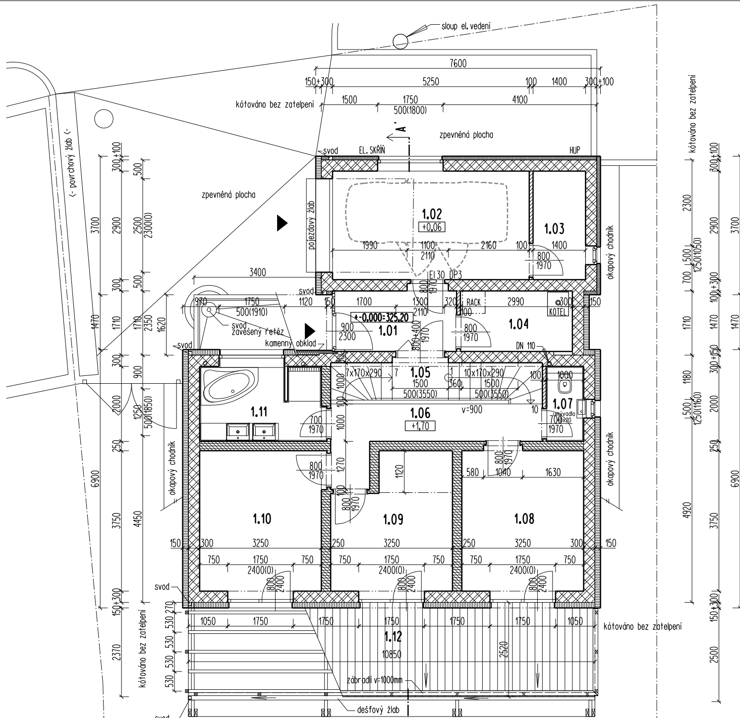
PŮDORYS 1.NP
