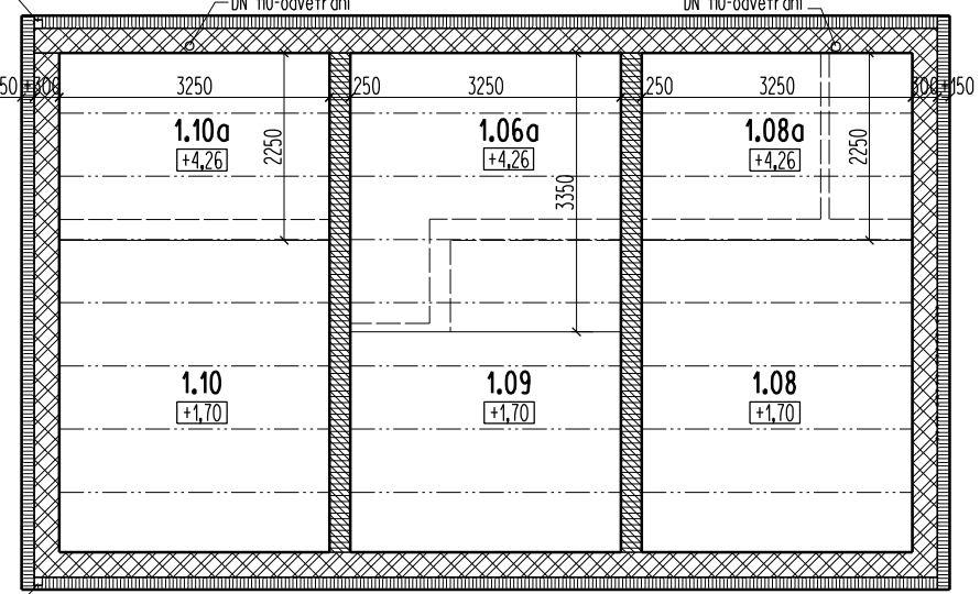
PŮDORYS 1.NP - GALERIE
